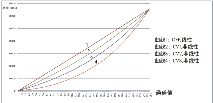
CURVE调光曲线图表
